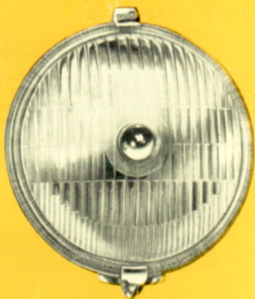
FOG LAMP (SFT 576) Part No. 57H 5314
